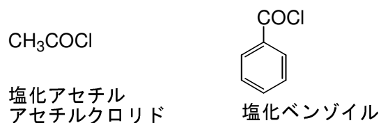
図 1. 塩化アシルの例.
