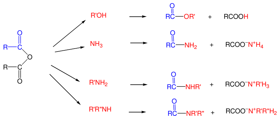
図1. 酸無水物とアルコール，アミン類との反応.
