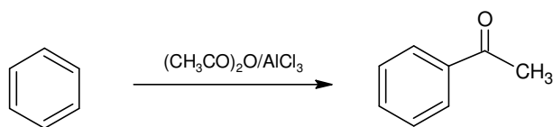
図2. 酸無水物を用いた Friedel-Crafts 反応の例.
