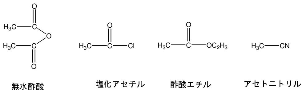
図 1. 酢酸のアシル体とニトリル.
