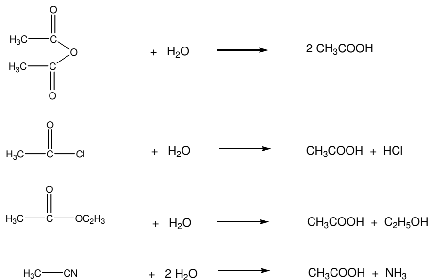
図 2. アシル体およびニトリルの加水分解.
