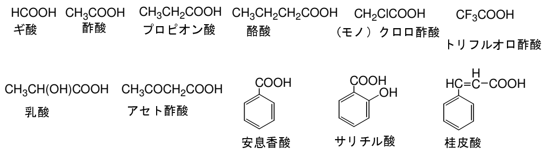
図 1. (モノ) カルボン酸の分子例.
