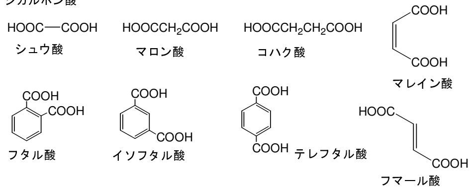
図 2. ジカルボン酸の分子例.
