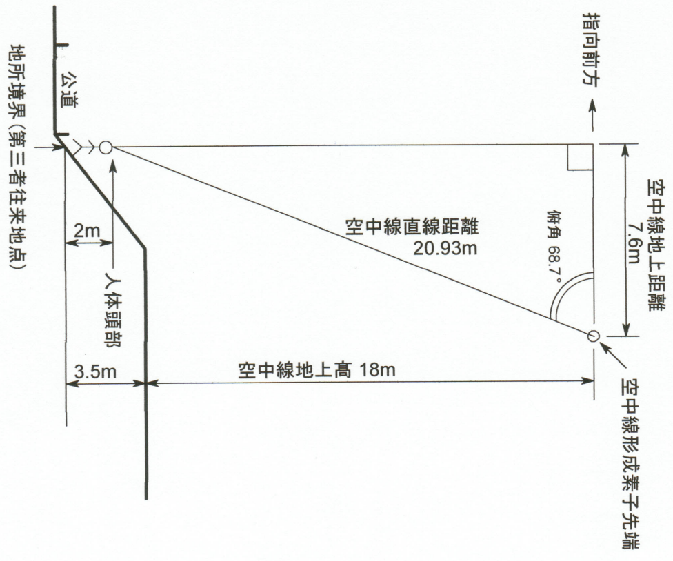
【俯角計算図】
